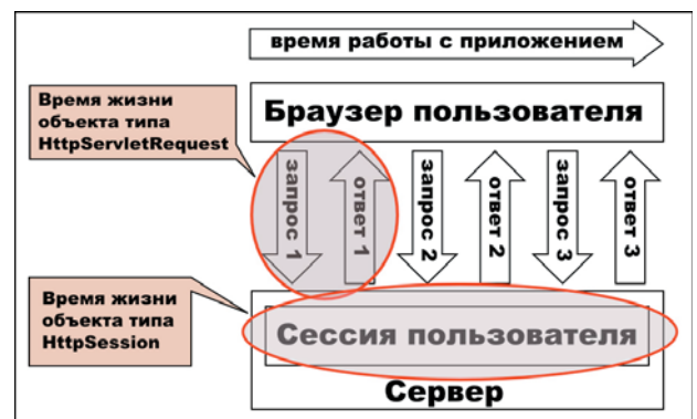
» (Рис. 1) Время жизни объектов HttpServletRequest и HttpSession .
