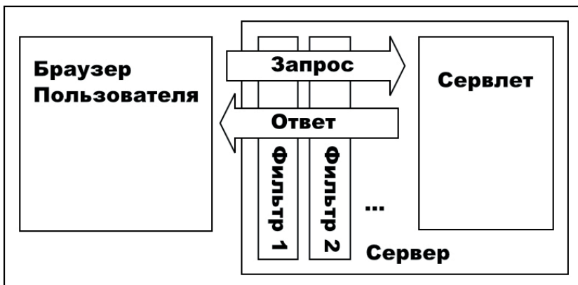
➤ (Рис. 3) Схема прохождения запроса через фильтры.
